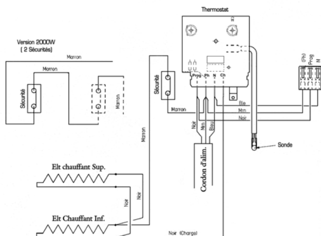
Schéma électrique
