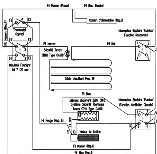
Schéma électrique
