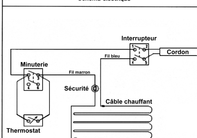
Schéma électrique
