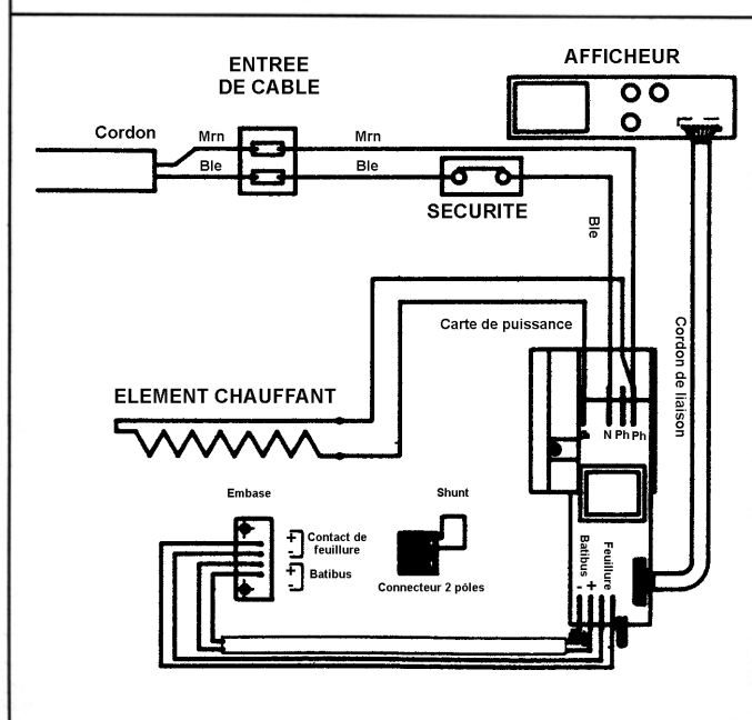
Schéma électrique
