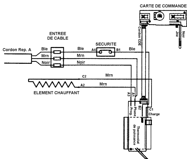
Schéma électrique
