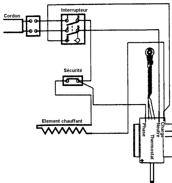
Schéma électrique
