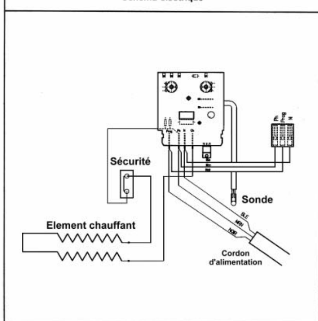
Schéma électrique
