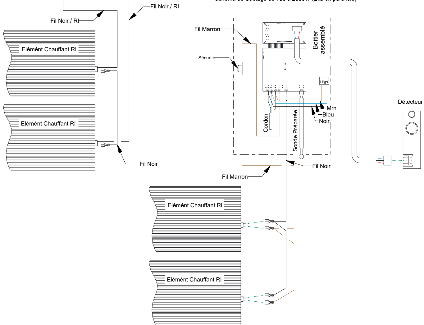
Schéma de Cablage de 750 à 2000W (Elts en parallèle)
