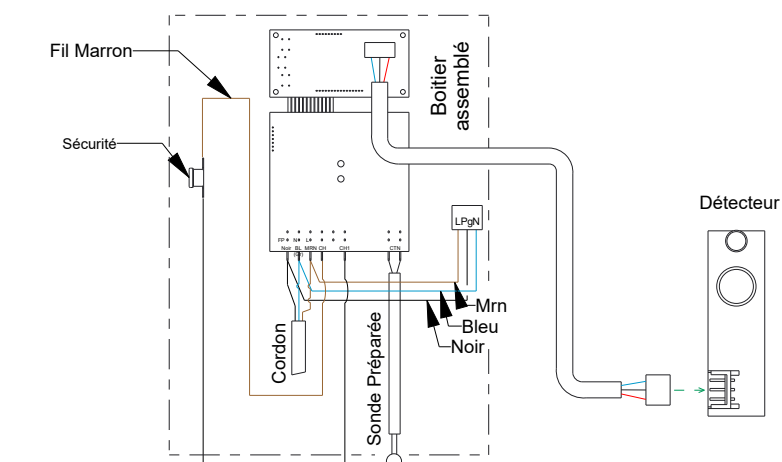
Schéma de Cablage 300 & 500W (Elts en série)
