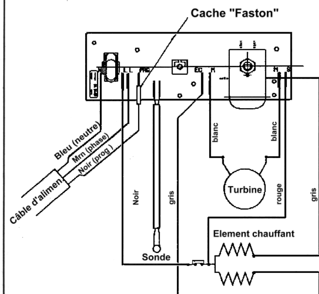
Schéma électrique
