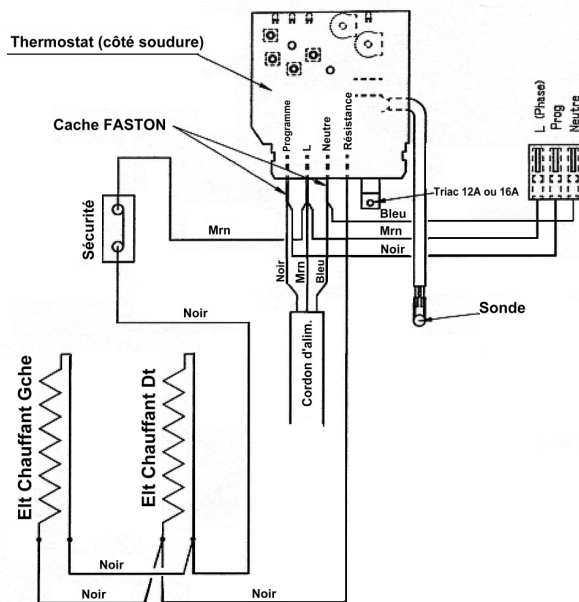
Schéma électrique
