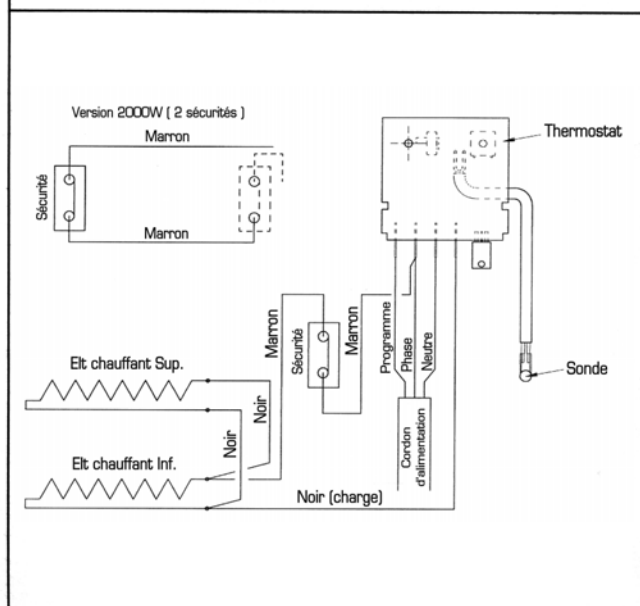
Schéma électrique
