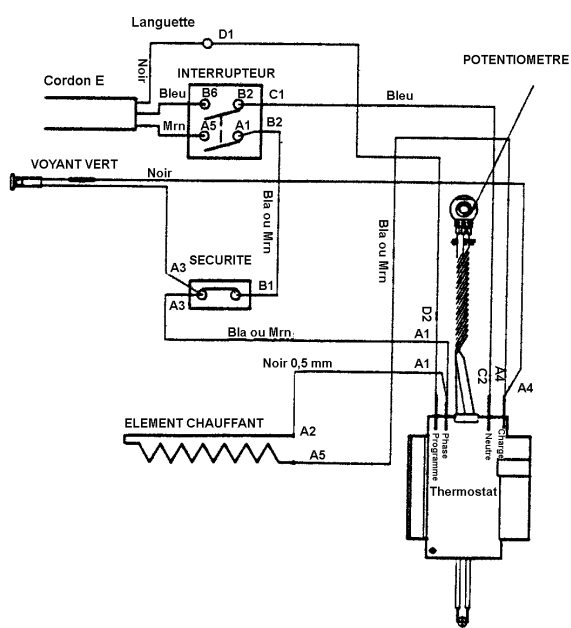
Schéma électrique
