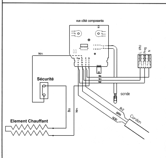
Schéma électrique
