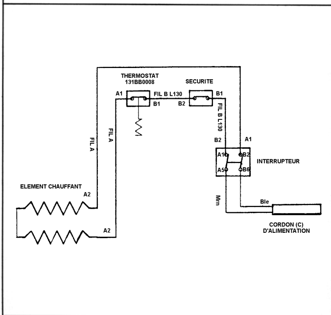
Schéma électrique
