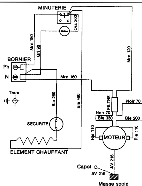
Schéma électrique
